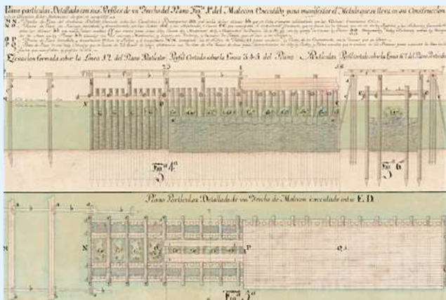
Figura 5. Fragmento del plano realizado por Antonio de Arebalo (firmaba con b) de 1777 donde muestra el detalle de la forma de construcción de la escollera bajo el agua.
